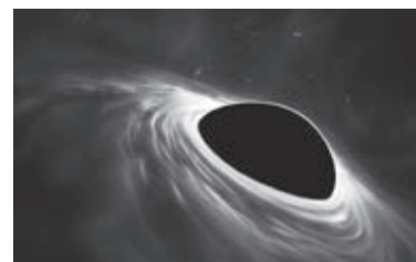
高速で回転する超巨大ブラックホールの姿(想像図) ©ESO, ESA/Hubble, M. Kornmesser
