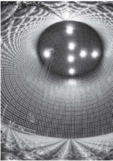
スーパーカミオカンデ 提供:東京大学宇宙線研究所 神岡宇宙素粒子研究施設
