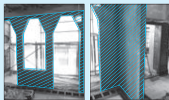
新たに設置した耐震補強壁(斜線部分)
