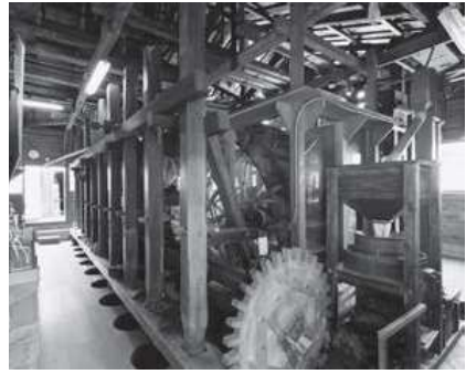
大沢の里水車経営農家の水車機構
