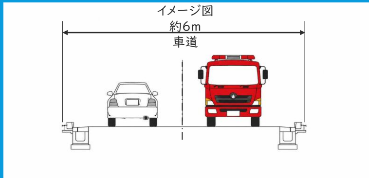
標準断面図(道路構造の概要)
