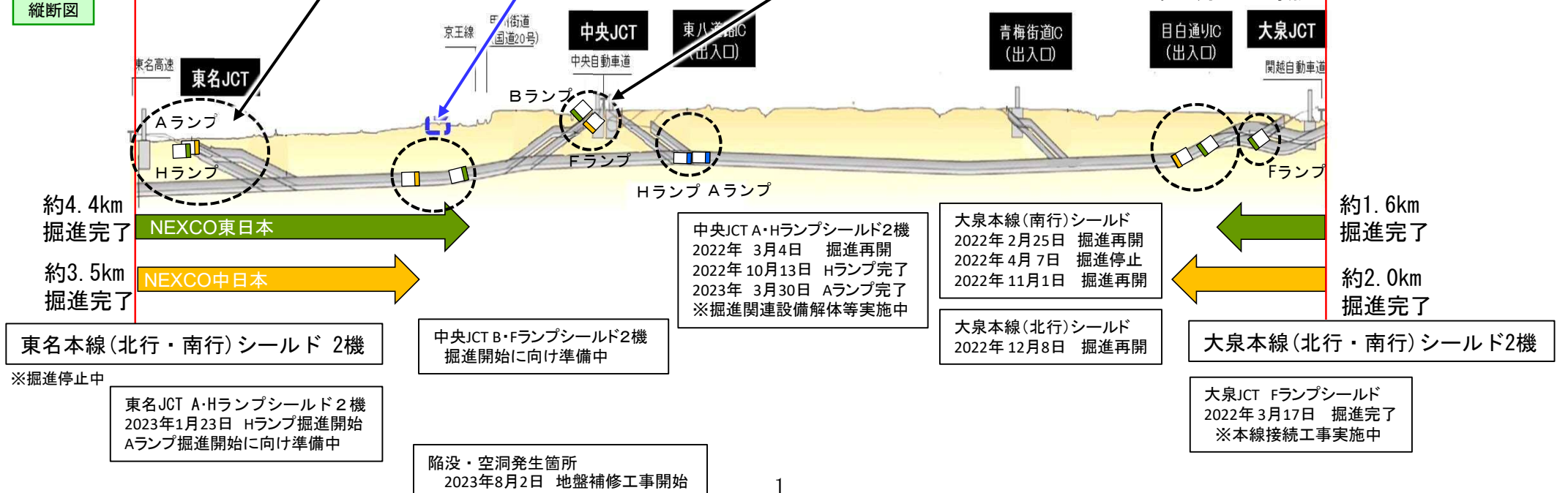
縦断面図
