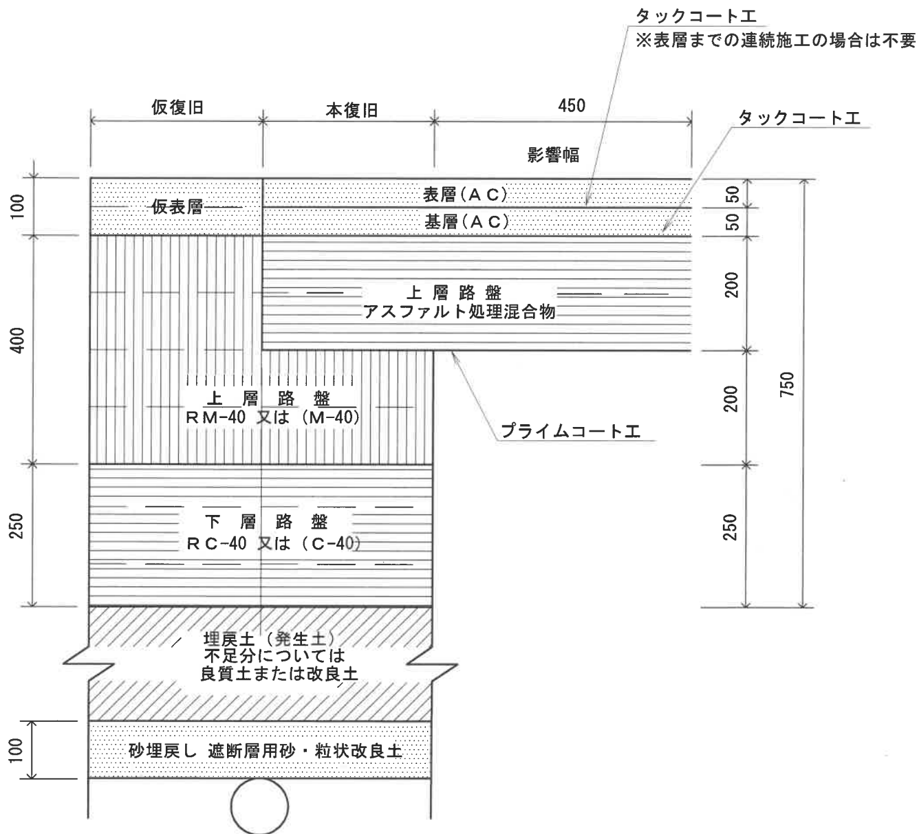
材 料 表
