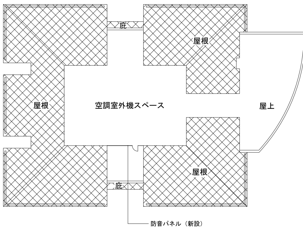
屋上平面図
