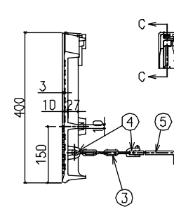
A-A断面図
