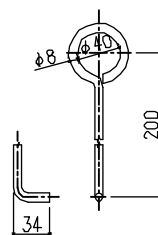
フック詳細図 S = 1 : 5
