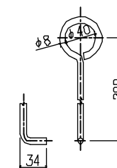
フック詳細図 S = 1 : 5
