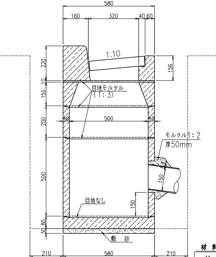
断面図
