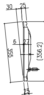
側面図
