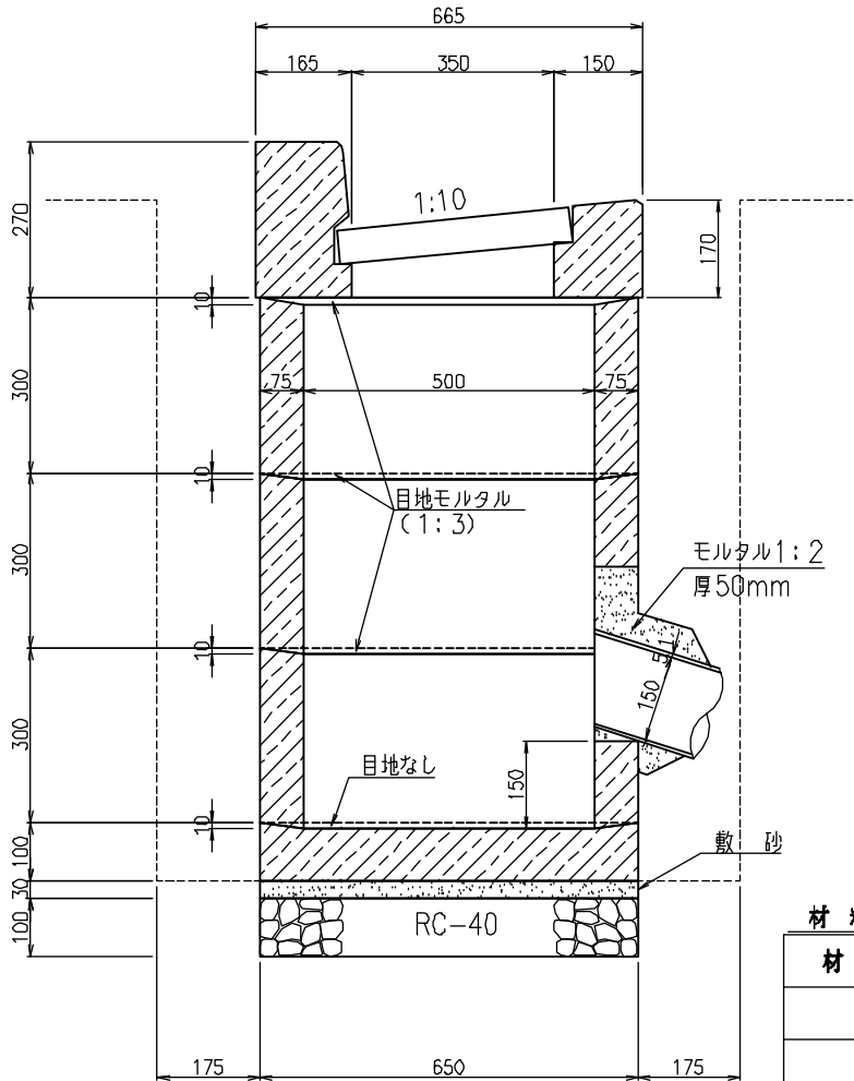
断面図
