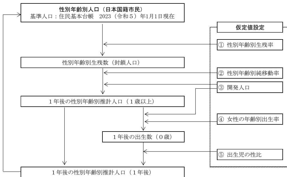
【図表8】コーホート要因法による推計の流れ（日本国籍市民）
