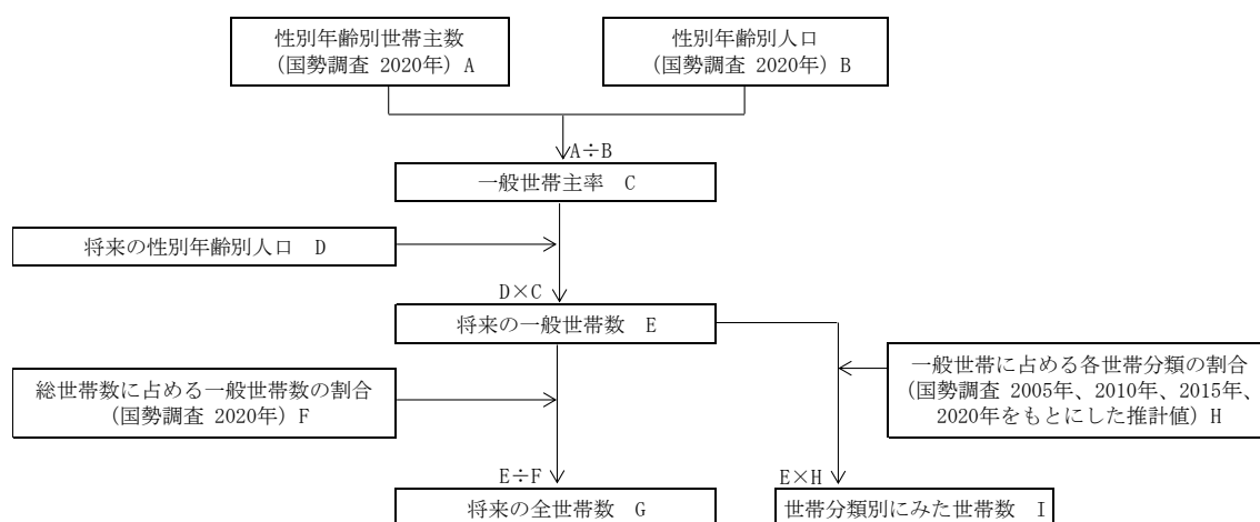
【図表 14】 将来世帯数の推計の流れ
