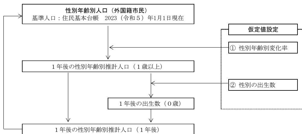
【図表9】 コーホート変化率法による推計の流れ（外国籍市民）
