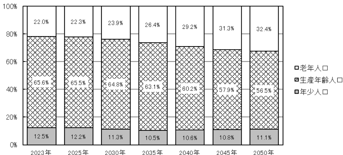
【図表12 続き】年齢3区分人口の将来推計
