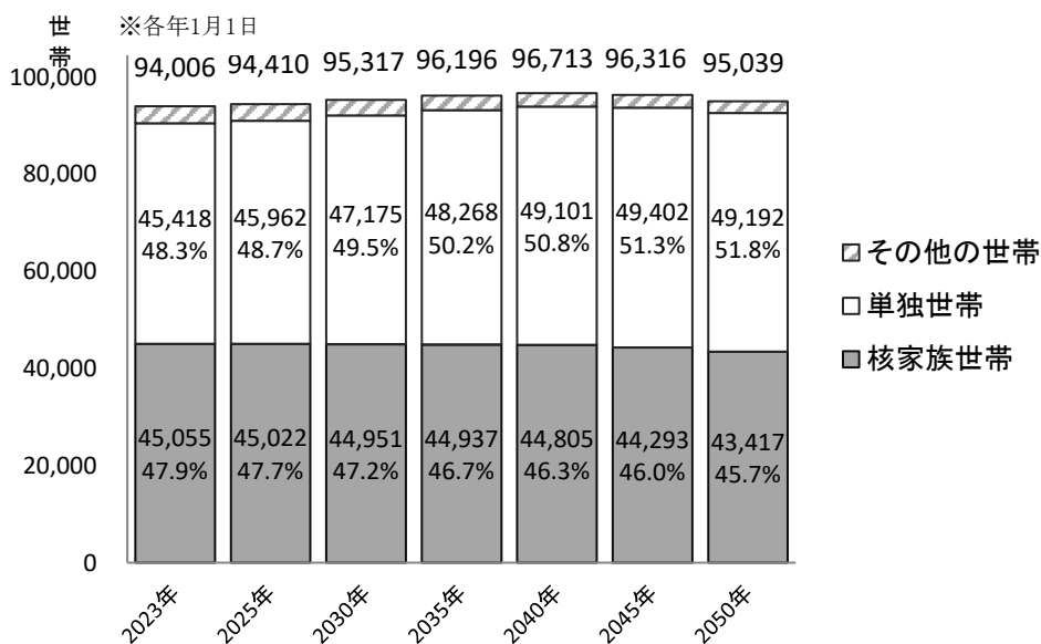
【図表 17】 将来の世帯分類別世帯数（グラフ）
