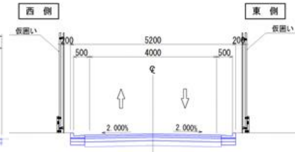
B-B断面 標準横断面(代替南北道路)
