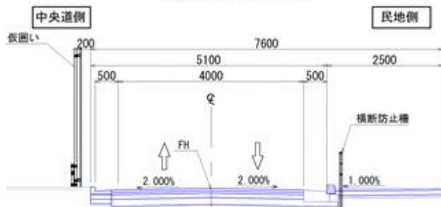
A-A断面 標準横断面(代替道路)
