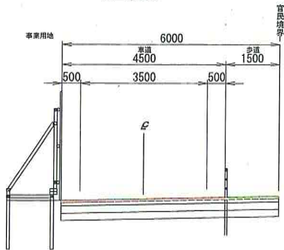
①-①断面
