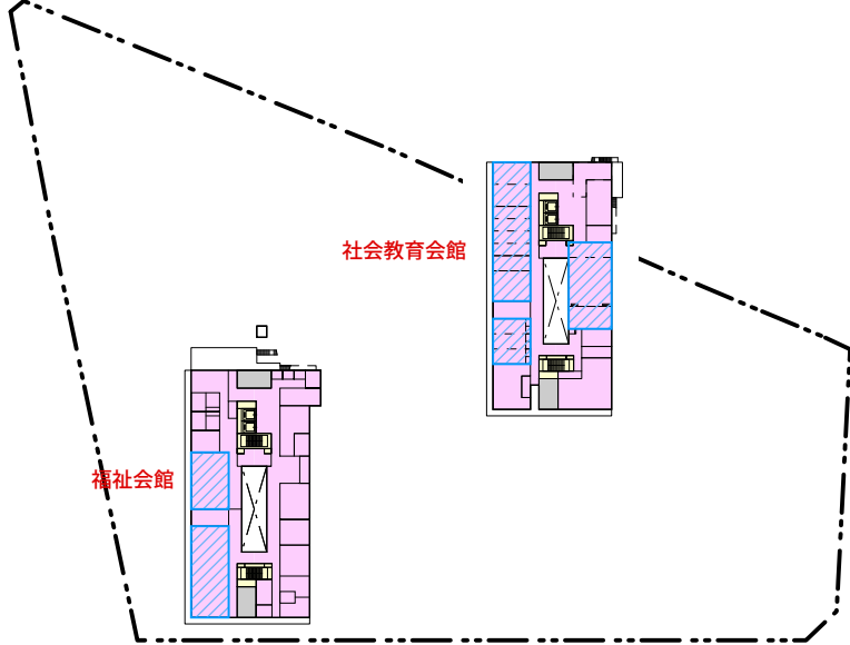
3, 4階平面図
