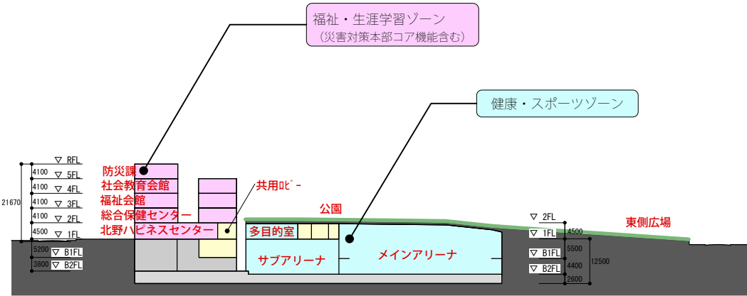
A-A' 断面図 1/1500
