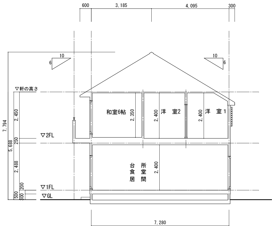
C-C' 断面図 1/100
