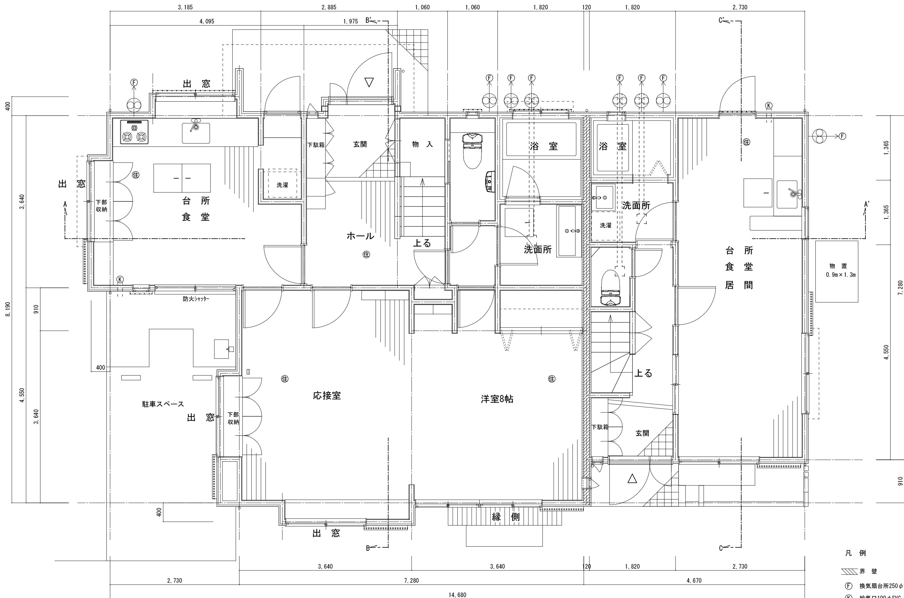
1階 平面図 1/50
