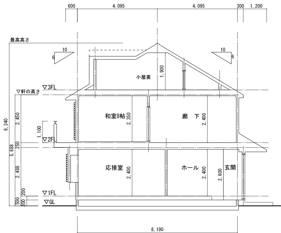
B-B' 断面図 1/100
