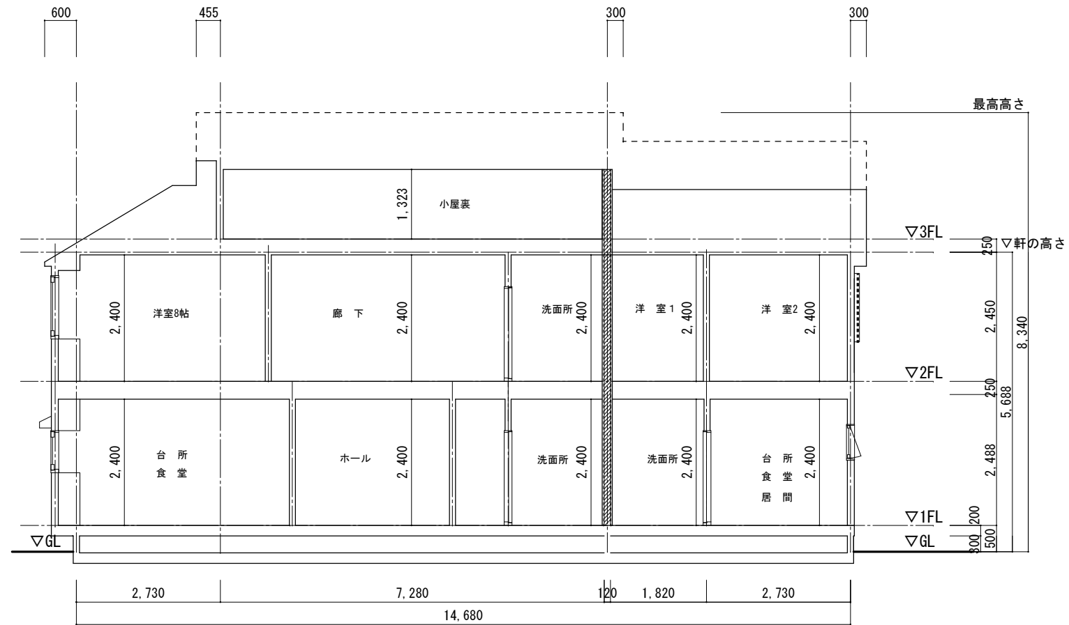
A-A' 断面図 1/100
