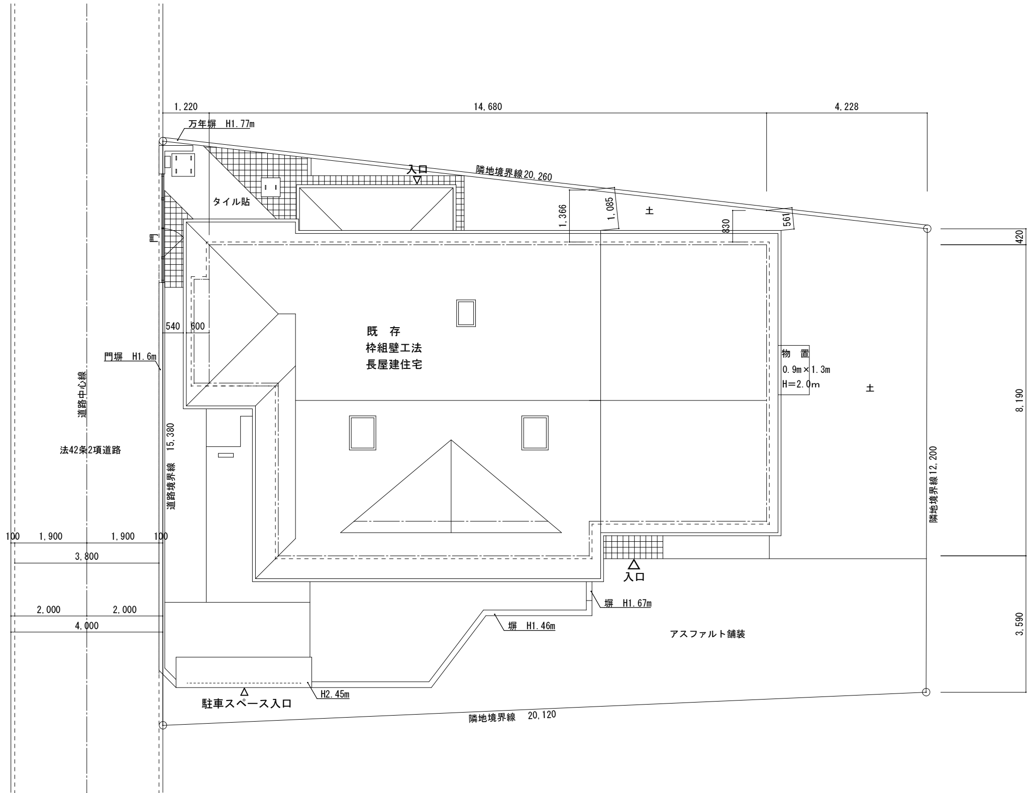
配置図 1/100
