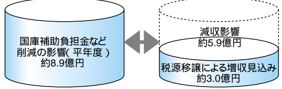
図2 「三位一体の改革」の三鷹市への影響 (平成19年度以降)
